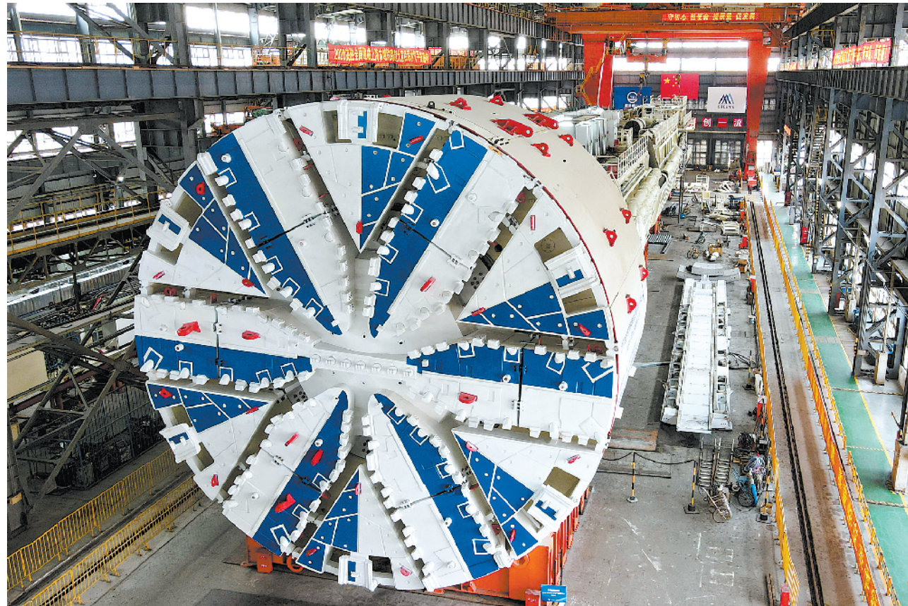
由隧道股份上海隧道工程有限公司自主研发的盾构机掘进与拼装同步技术近日试验成功。应用推拼同步技术,可实现掘进与拼装并联作业。图为上海隧道机械制造分公司车间内的“骠跃”盾构机。新华社发
